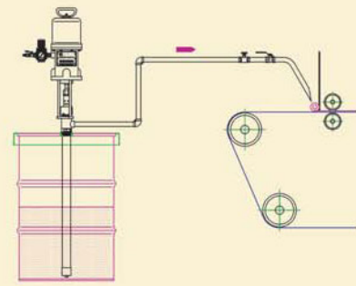
Spraying 噴塗作業
