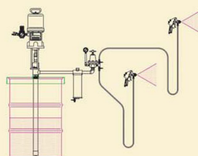
Spraying 噴塗作業
